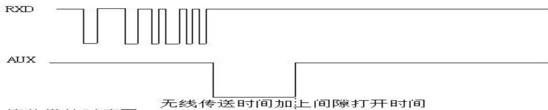
接收模块时序图：
